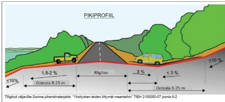
Joonis 1. Ristumiskoha pikikallete kujundamine
